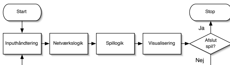
Figur 4.1: Flow chart for et eksemplarisk action spil
