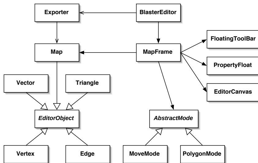
Figur 11.3: Klasserne i editoren og deres sammenhæng
