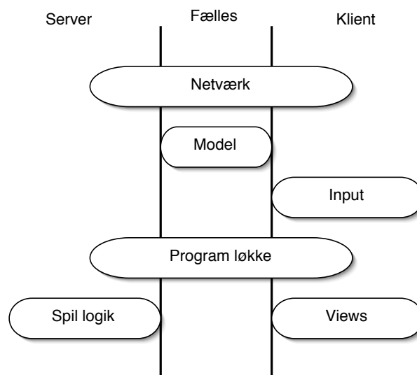
Figur 7.2: Oversigt over hvor delene hører til
