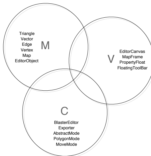
Figur 11.2: Klasserne indelt i MVC
