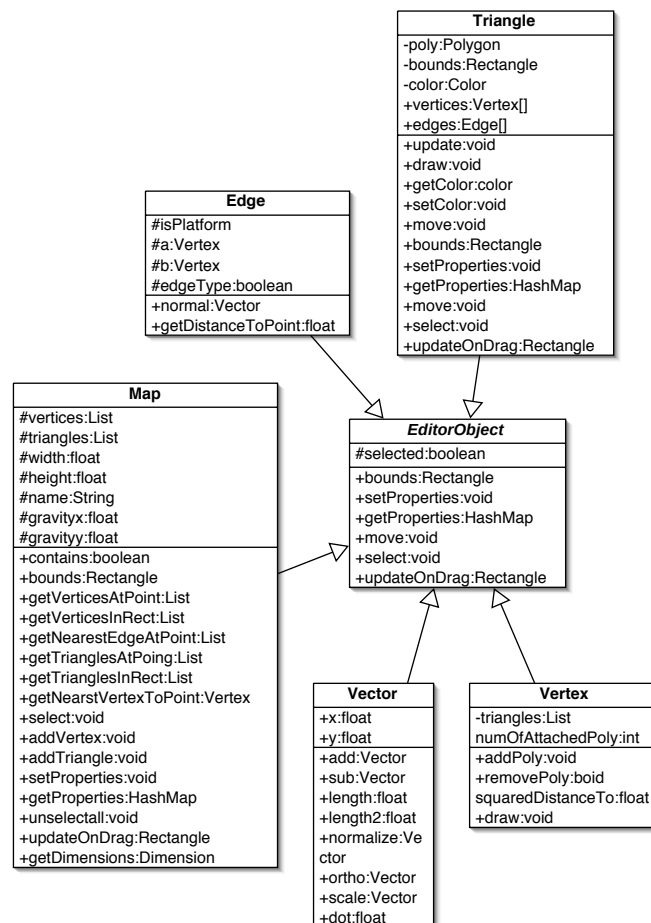
Figur 12.2: Klasserne i model-pakken
