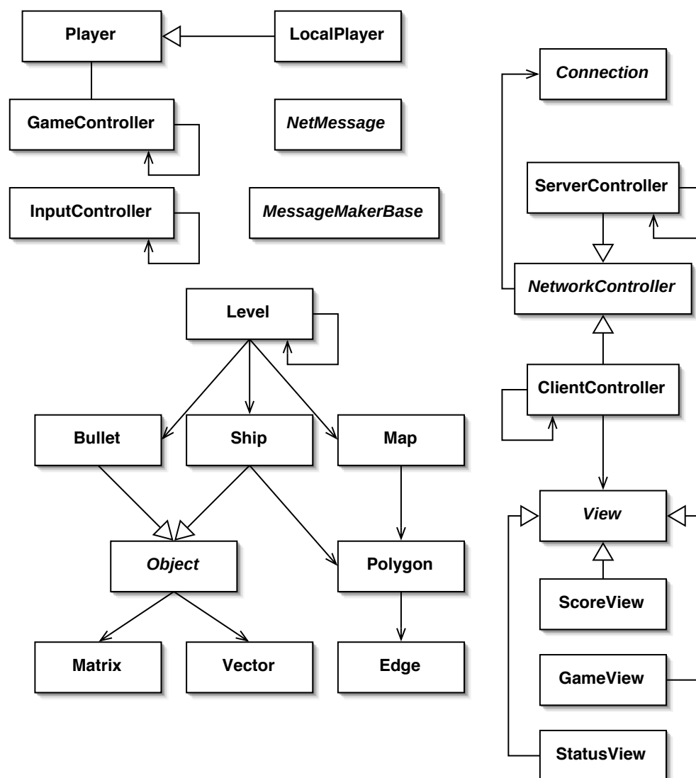
Figur A.1: Samlet oversigt over klient og server
