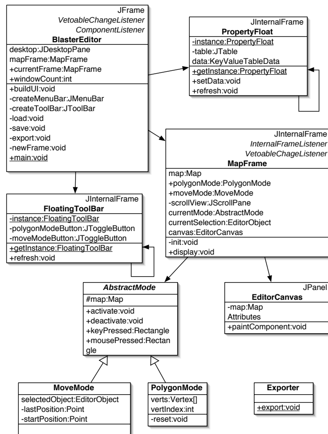
Figur 12.1: Klasserne i ui-pakken
