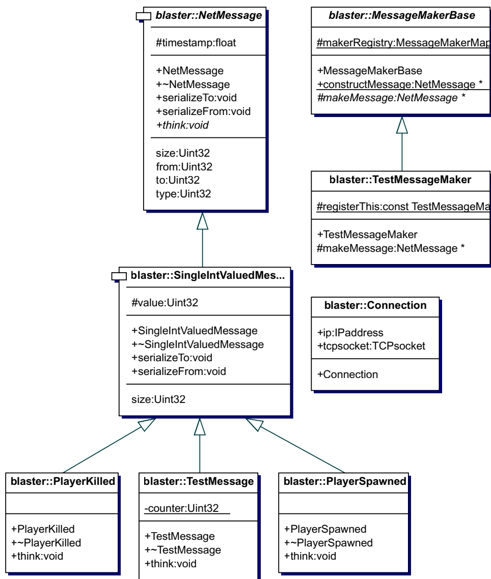
Figur A.4: UML diagram over netværks model delen
